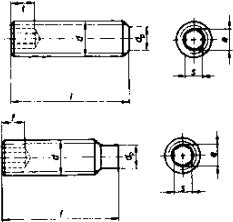
DIN 913 Kegelkuppe
